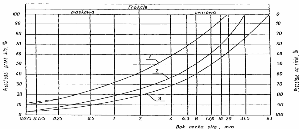
Rysunek 1. Pole dobrego uziarnienia kruszyw przeznaczonych na podbudowy wykonywane metodą stabilizacji mechanicznej 1-2 kruszywo na podbudowę zasadniczą (górną warstwę) lub podbudowę jednowarstwową
